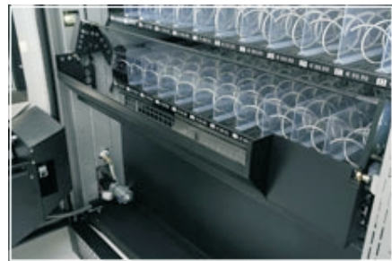
Warenlift (Glasflaschen usw.)
